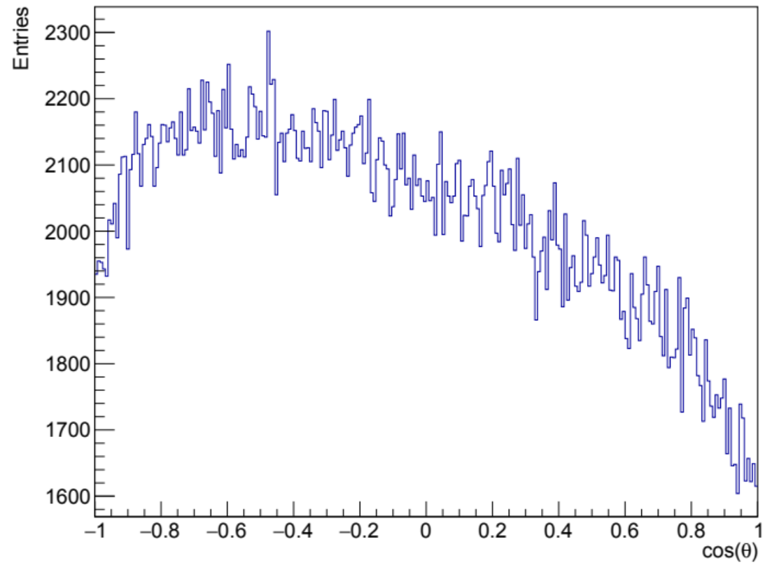
\cos(\theta) ( \bar{t} -Quark und W^- -Boson nach Selektion aus der Teilchenliste)
