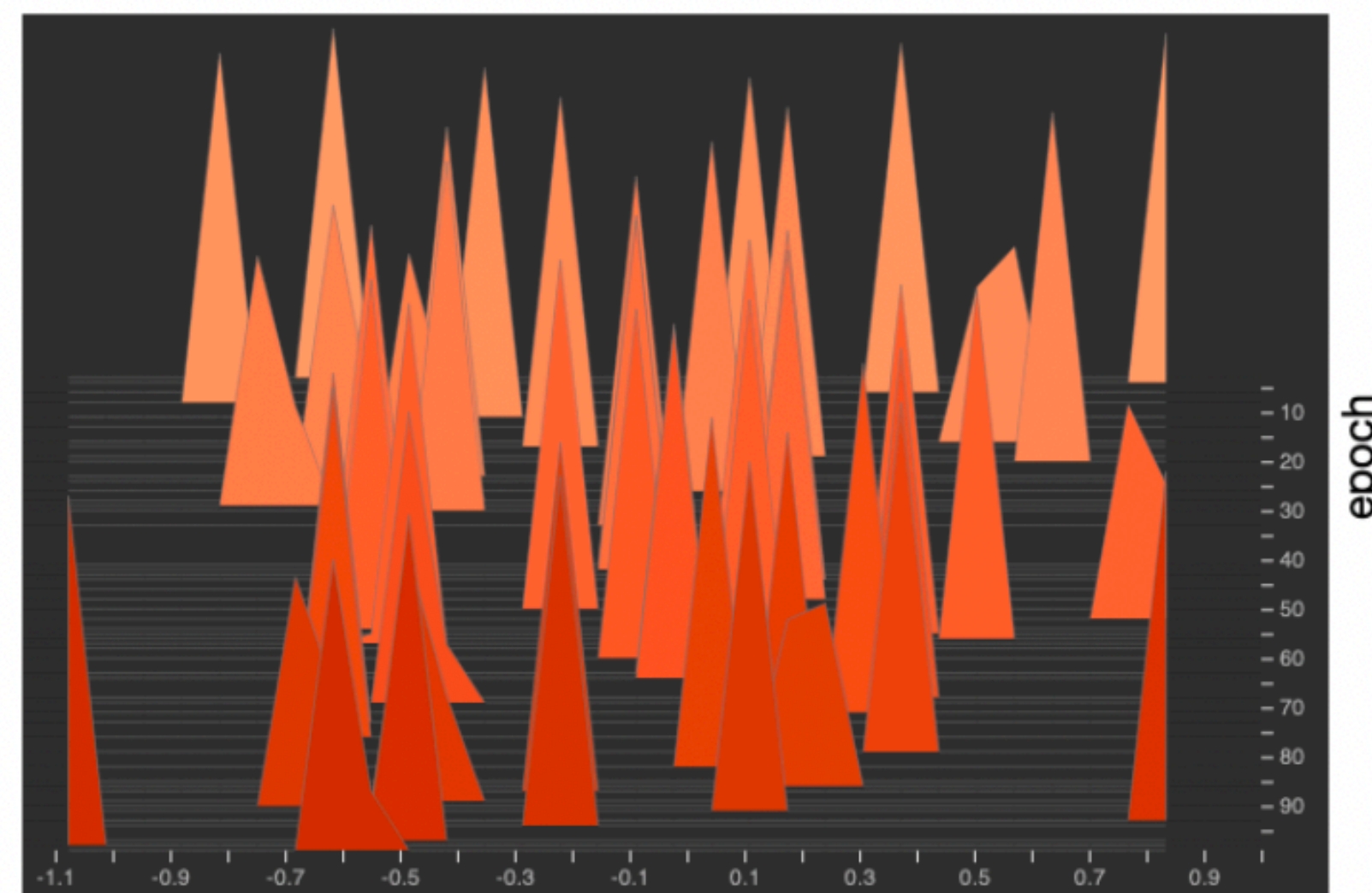
bias gradient
